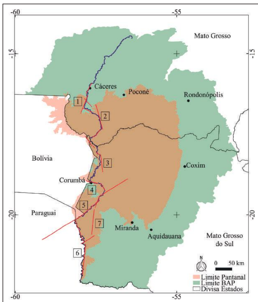
Figura 5 Lineamentos estruturais coincidentes com o rio Paraguai. As mudanças de direção que ocorrem no rio Paraguai estão diretamente relacionadas à presença de estruturas lineares, conforme indicado na figura. Ab'Saber (1988) já havia mencionado que a mudança desse rio foi induzida por tectônica. O ponto 7 refere-se ao atual curso do rio Nabileque, descrito por Kuerten & Assine (2011) como paleocanal do rio Paraguai.
