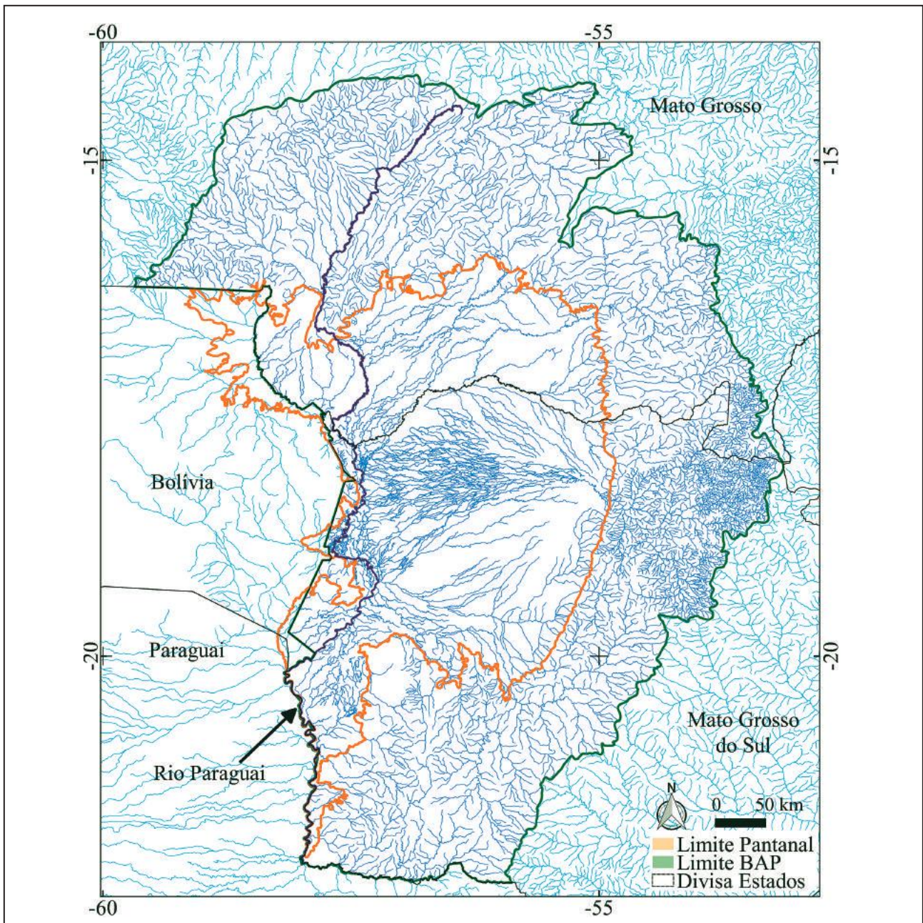
Figura 4 Na região de planalto, o padrão da drenagem da BAP (limite em verde) diferencia-se consideravelmente da drenagem da planície pantaneira (em laranja), onde a mesma se apresenta de forma distributária. Nota-se forte assimetria da bacia, pois os afluentes da margem esquerda do Rio Paraguai distribuem-se de maneira diferenciada quando comparados aos da margem direita.
