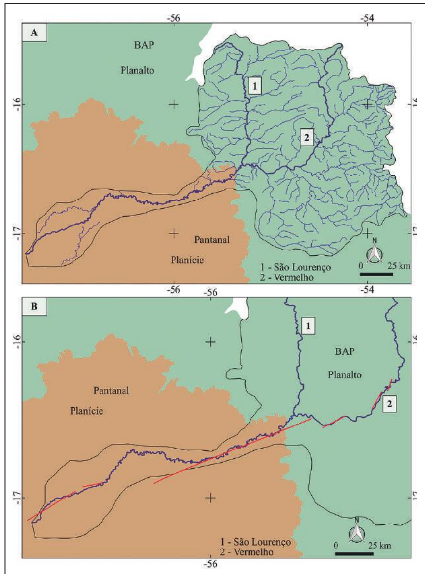
Figura 13 A. Bacia Hidrográfica do rio São Lourenço (ponto 1) e seu principal afluente, o rio Vermelho (ponto 2). Ao adentrar a planície, a bacia sofre um “estrangulamento” pelos planaltos (Corradini, 2011) e o rio São Lourenço passa a ser meandrante. B. O rio São Lourenço, a partir do momento que adentra a planície pantaneira, corre encaixado, com padrão meandrante.
