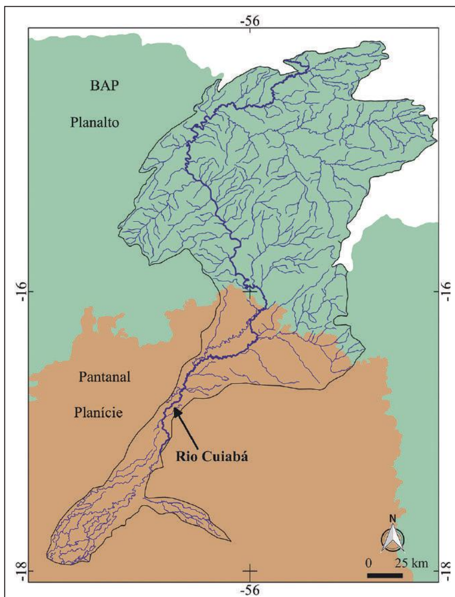
Figura 14 A Bacia Hidrográfica do rio Cuiabá, assim como a do rio São Lourenço, sofre um “estrangulamento” ao adentrar o Pantanal, apresentando também assimetria.
