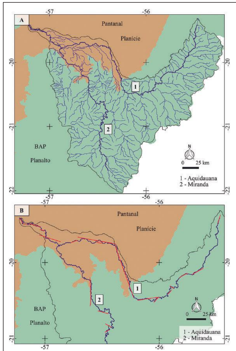
Figura 9 A. Drenagem da Bacia Hidrográfica do rio Miranda. Sua área no planalto é de aproximadamente 86%, onde apresenta padrão tributário e assimétrico na porção norte. No ponto 1 tem-se o rio Aquidauana e no ponto 2 o rio Miranda. A assimetria mostra-se presente no trecho do planalto do rio Aquidauana. B. O rio Aquidauana (ponto 1) é quase inteiramente condicionado por estruturas, principalmente no trecho em que corre dentro do Pantanal, além de apresentar padrão assimétrico.
