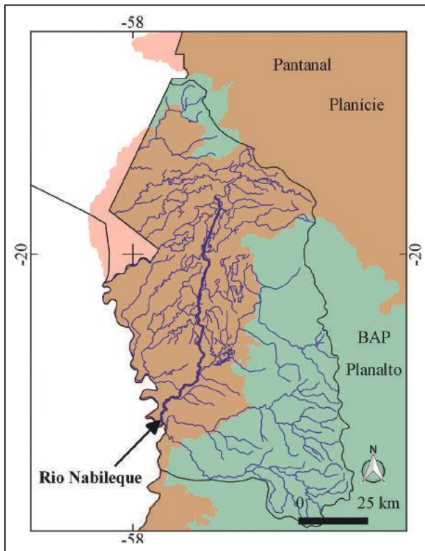
Figura 10 Bacia Hidrográfica do rio Nabileque. A maior parte da Bacia Hidrográfica do rio Nabileque situa-se na planície pantaneira. Nessa região, o padrão é distributário.
