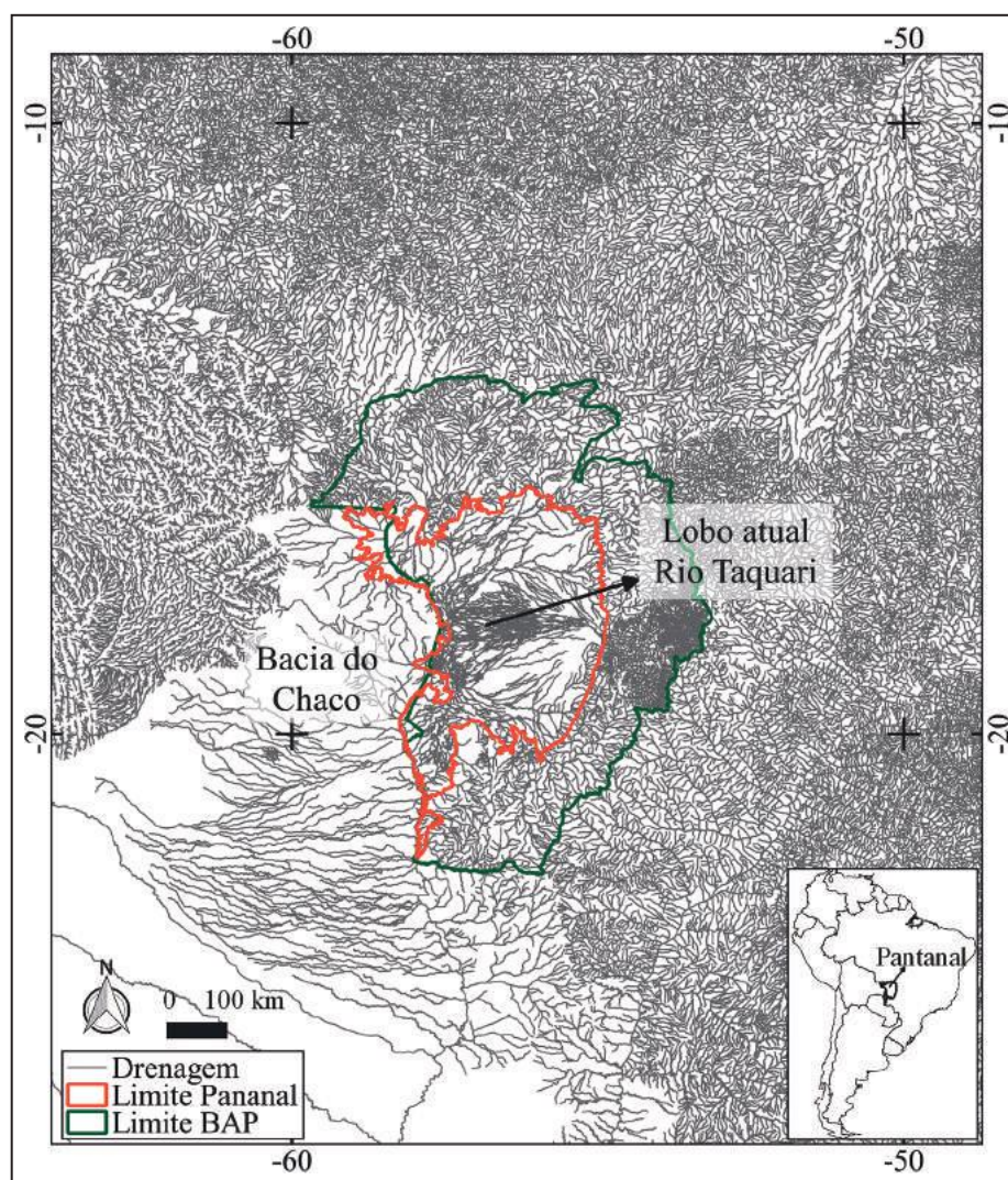
Figura 3 A rede hidrográfica do Pantanal quando comparada à malha hidrográfica do entorno destoa-se intensamente. As baixas declividades somadas à baixa precipitação e alta permeabilidade do substrato conferem um padrão único ao Pantanal e completamente diferente do planalto circundante.
