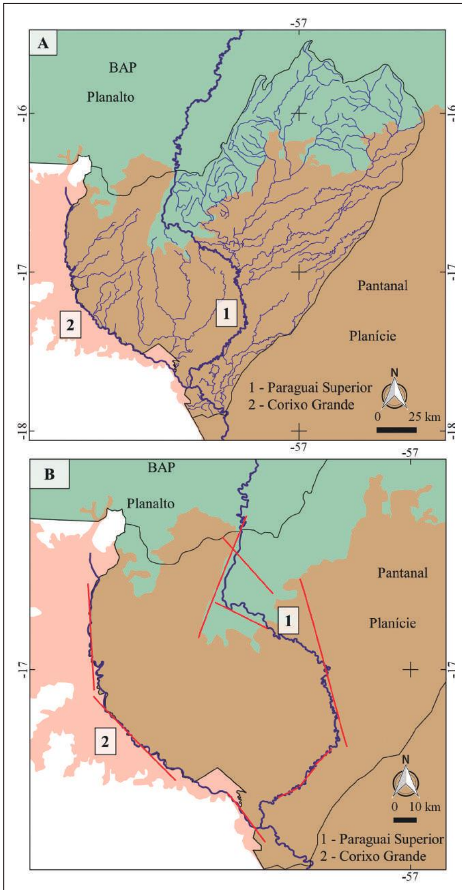
Figura 16 A. Bacia Hidrográfica do Paraguai Superior e seu padrão de drenagem assimétrico. O ponto 1 indica o trecho do rio Paraguai dentro da bacia e o ponto 2 indica o rio Corixo Grande. B. O rio Paraguai (ponto 1) é condicionado quase inteiramente por estruturas, assim como o rio Corixo Grande (ponto 2).
