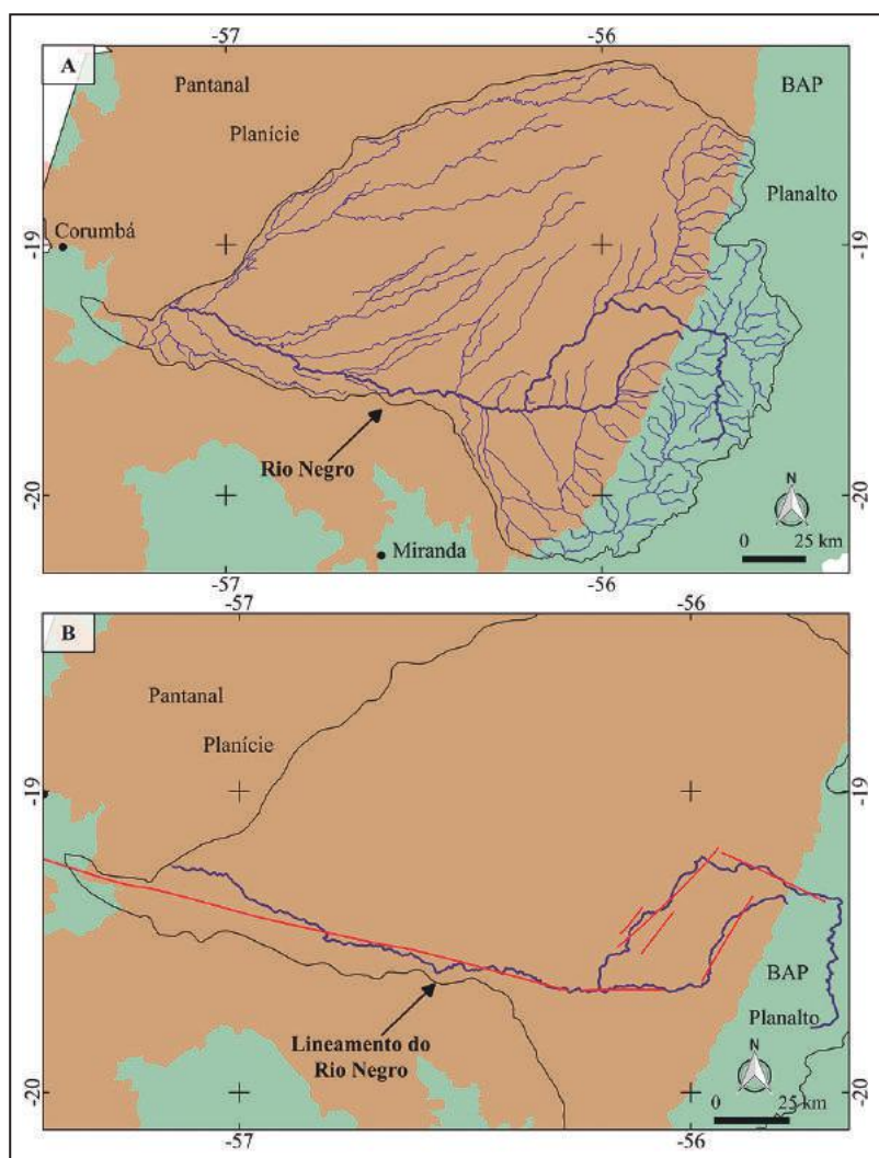
Figura 8 A. A maior parte da Bacia do rio Negro encontra-se dentro do Pantanal, caracterizada por padrão radial (região do leque do rio Taquari). Também é uma bacia assimétrica, pois apresenta diferenças quando analisada no planalto e na planície. B. Lineamentos estruturais que condicionam o rio Negro. O ponto 1 indica o Lineamento do rio Negro descrito por Mendes (2008), o qual condiciona o rio e é também o limite da área com a presença das lagoas da região da Nhecolândia.
