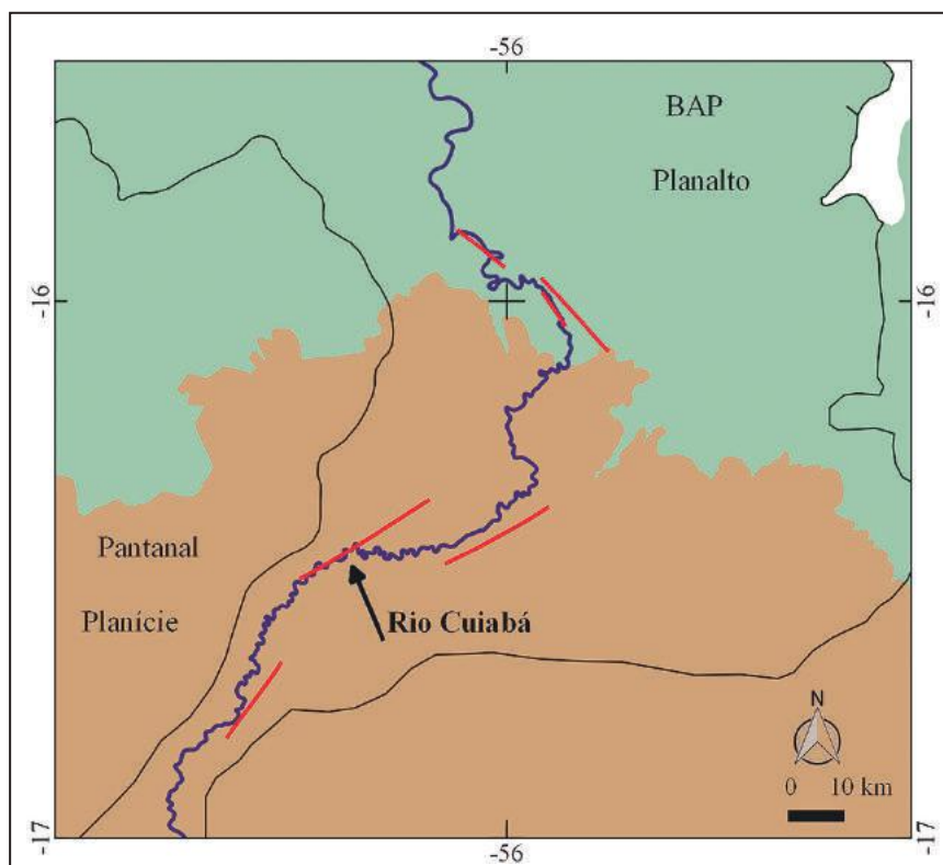
Figura 15 O rio Cuiabá, à medida que flui para o rio Paraguai, mostra-se confinado em estruturas, tornando-se meandrante na planície pantaneira.
