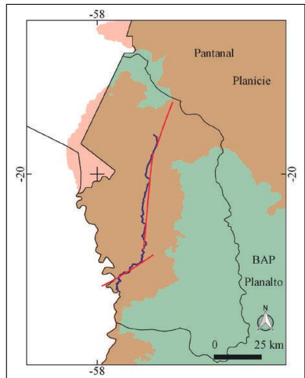
Figura 11 O rio Nabileque flui na direção NS, onde anteriormente corria o rio Paraguai. Também é condicionado por lineamentos estruturais e apresenta-se assimétrico.
