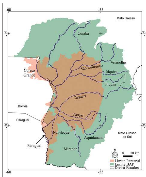
Figura 1 Localização dos principais rios que compõem o Pantanal.
