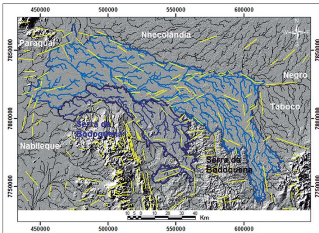
Figura 7 Delimitação dos Pantanaís de Aquidauana (azul escuro) e Miranda-Abobral (azul claro) por meio da comparação de malha hidrográfica e fotolineamentos estruturais (em amarelo).
