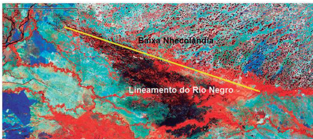
Figura 5 Imagem Landsat TM na composição falsa-cor RGB (457) mostrando a diferença na estrutura da paisagem a norte e sul do Lineamento do Rio Negro, assim denominado por Mendes et al. (2006).
