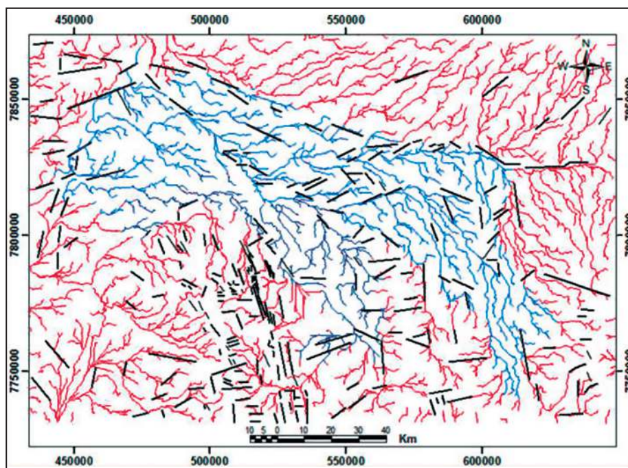
Figura 6 Sobreposição de lineamentos (preto) e das linhas de escoamento superficial (obtidas do SRTM), em azul claro o Pantanal de Miranda-Abobral e em azul escuro o Pantanal de Aquidauana. Em vermelho, outros pantanais ou fora do contexto Pantanal.
