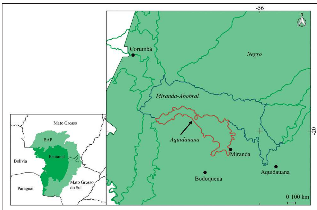
Figura 2 Localização dos Pantanaís de Miranda-Abobral (em azul) e Aquidauana (em vermelho); a delimitação de Pantanal utilizada é a de Mioto et al. (2012).
