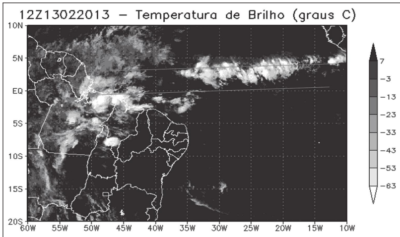
Figura 2 Imagem de satélite com dados de temperatura de brilho ( ^{\circ}\text{C} , tons de cinza) ilustrando a banda dupla da ZCIT no dia 13/02/2013 às 12 UTC. A posição da BP e da BD foi traçada em todo o domínio devido à identificação nos campos atmosféricos (umidade relativa e convergência de massa em 925 hPa) mostrados na Figura 3.
