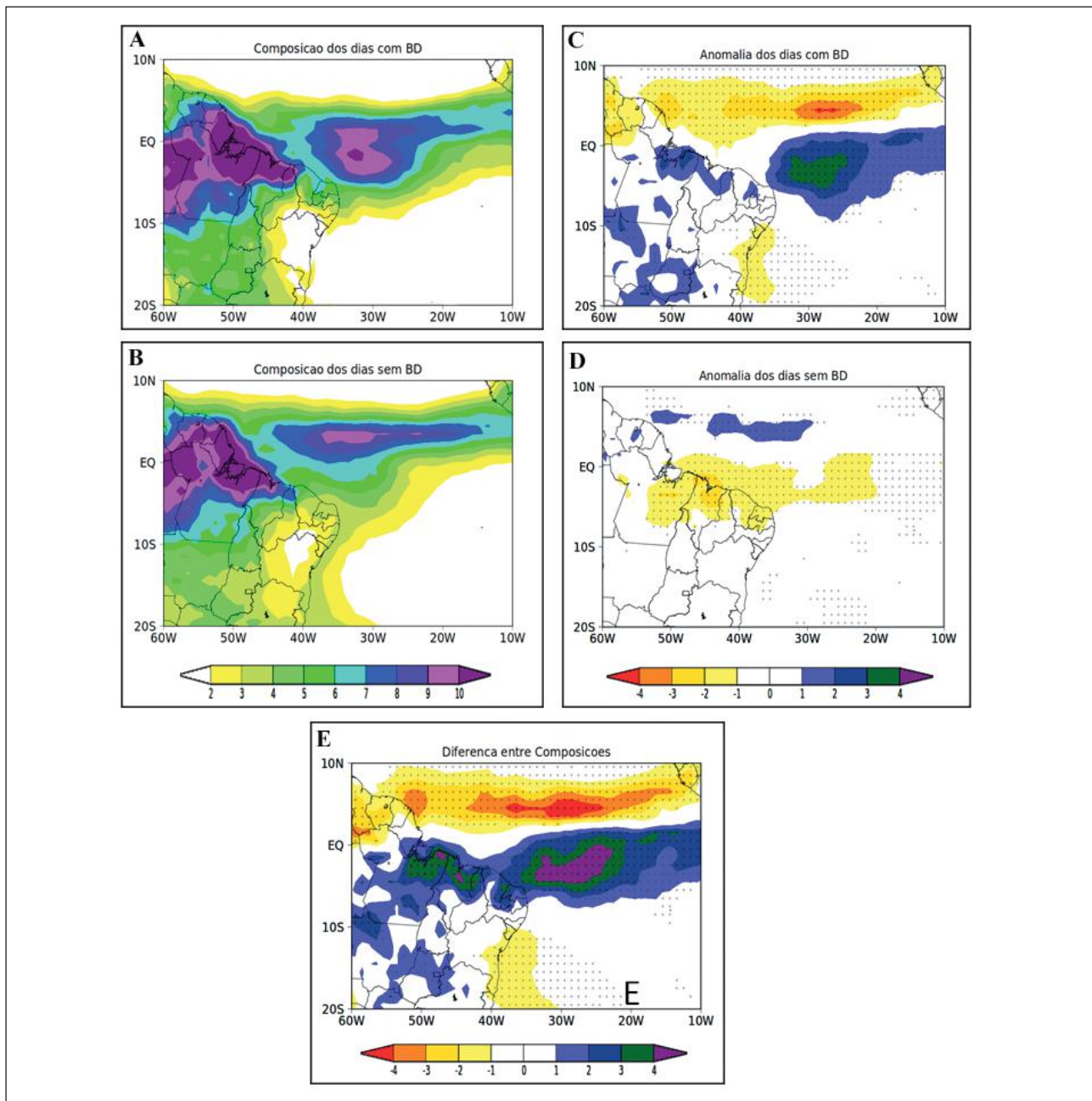
Figura 8 Similar à Figura 6, mas para o campo de precipitação ( \text{mm dia}^{-1} ) sobre o oceano Atlântico Tropical.
