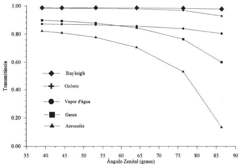
Figura 5 - Transmitâncias dos constituintes atmosféricos em função do ângulo zenital
