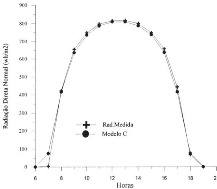
Figura 1c - Radiação Direta Medida e Estimada pelo Modelo C, em 9/6/92
