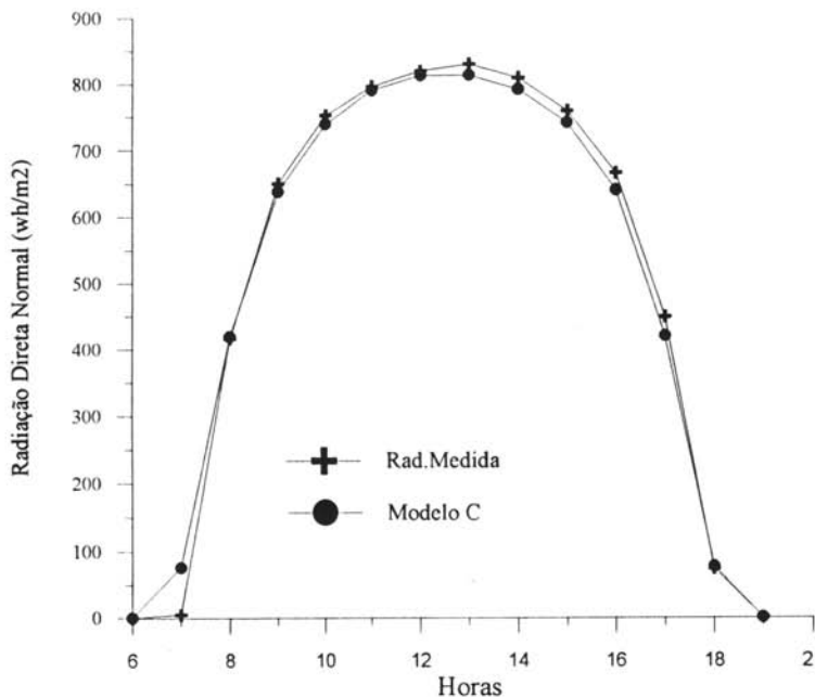
Figura 1b - Radiação Direta Medida e Estimada pelo Modelo C, em 7/6/92
