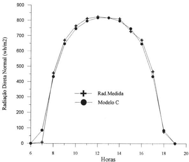
Figura 1a - Radiação Direta Medida e Estimada pelo Modelo C, em 28/5/92
