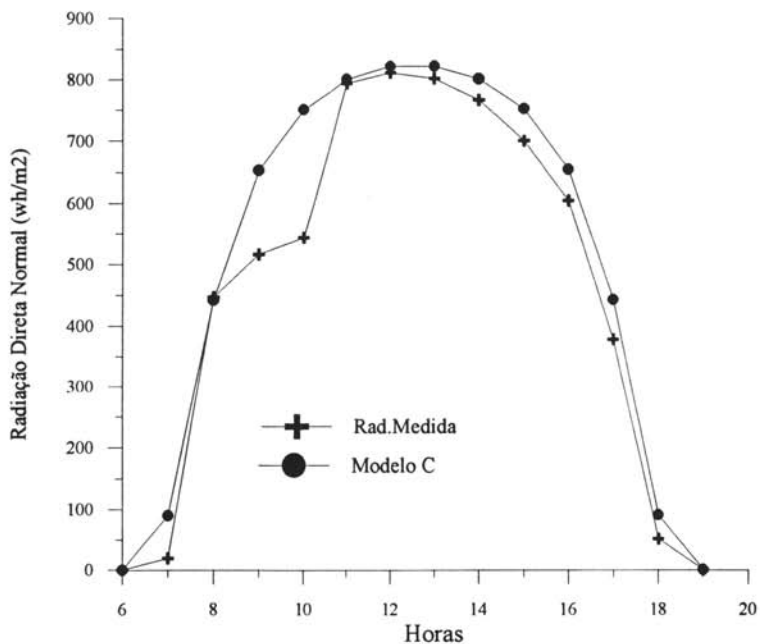
Figura 2a - Radiação Direta Medida e Estimada pelo Modelo C, em 23/5/92
