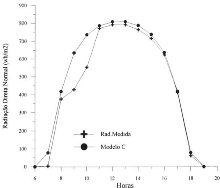
Figura 2c- Radiação Direta Medida e Estimada pelo Modelo C, em 05/6/92
