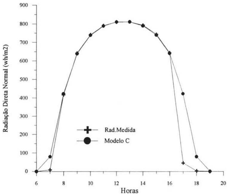
Figura 2b- Radiação Direta Medida e Estimada pelo Modelo C, em 02/6/92
