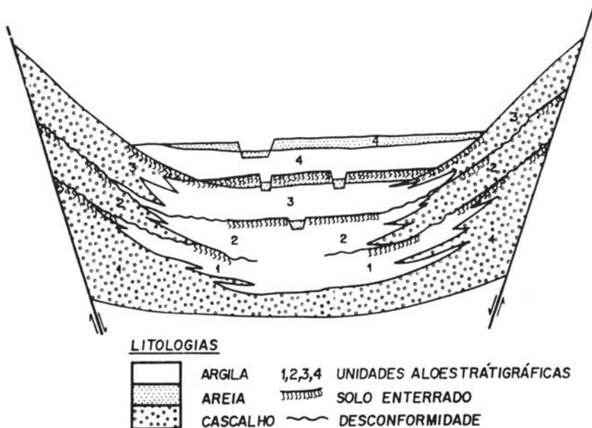
Figura 1: Esquema ilustrativo da utilização da perspectiva aloestratigráfica e da relação aloestratigrafia-litoestratigrafia: quatro unidades aloestratigráficas superpostas, definidas por discontinuidades lateralmente traçáveis (desconformidades e solos enterrados), reunindo duas classes litológicas principais (uma ou duas unidades litoestratigráficas). (Modificado de N.A.S.C.N., 1983)
