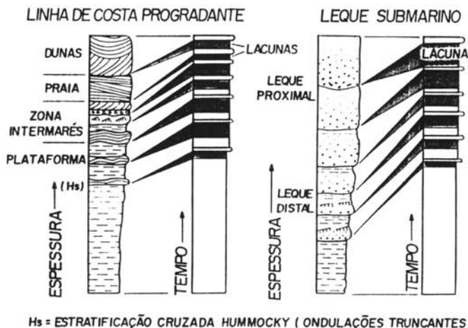
Figura 2: Perfis comparativos da espessura do registro sedimentar e do tempo envolvido em sua construção (in Dott, 1983). Considerável espaço de tempo é representado por
