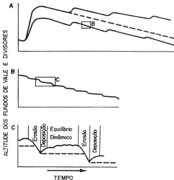
Figura 3: Ciclo geomorfológico de Davis (linha tracejada) modificado para ajustar-se ao conceito de erosão episódica, associada a rompimentos de estados de equilíbrio em
