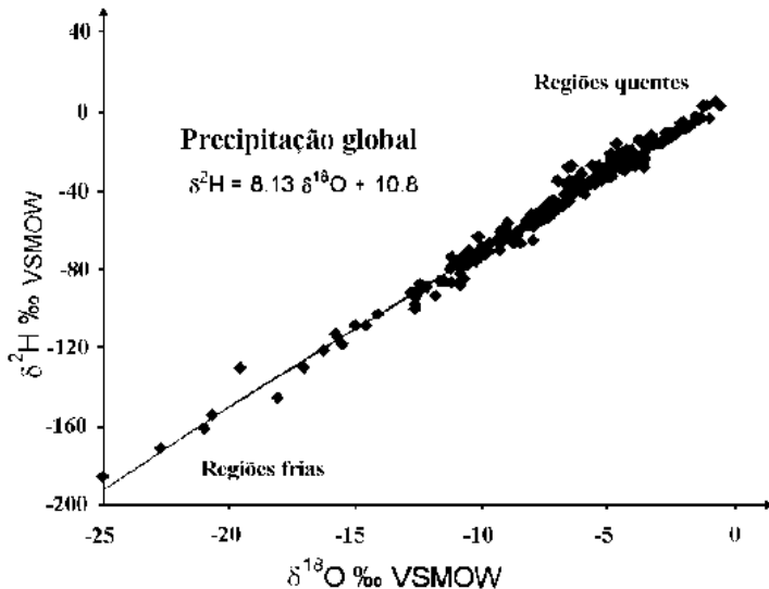
Figura 1 Reta meteórica mundial mostrando a relação entre \delta^{18}\text{O} e \delta^2\text{H} na chuva. Os valores mais enriquecidos em \delta^{18}\text{O} e \delta^2\text{H} são representativos da precipitação nas regiões mais quentes do mundo (modificado de Clark & Fritz, 1997).
