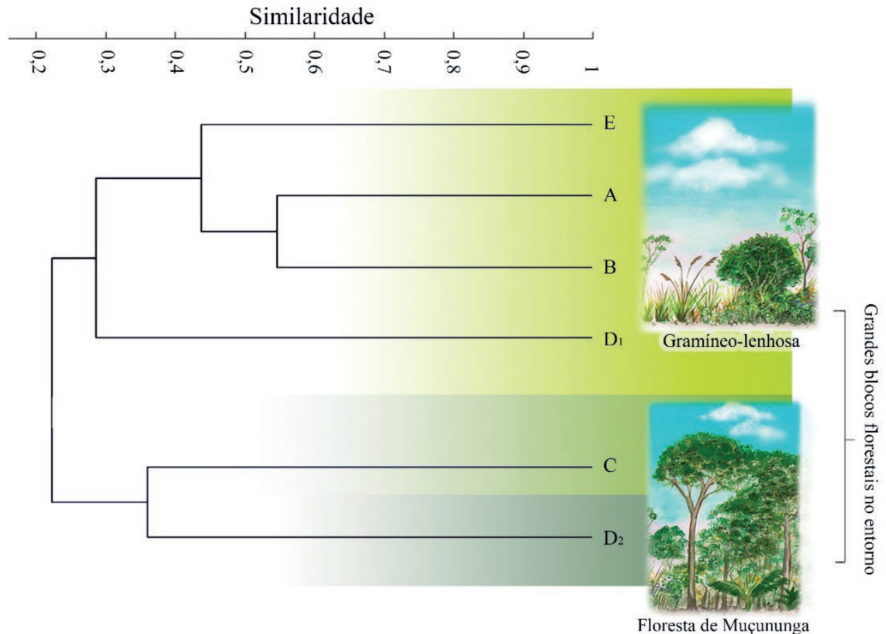
Figura 5. Dendrograma originado da análise de agrupamento pareado igualmente ponderado (UPGMA), que compara a similaridade entre as cinco áreas de muçunungas avaliadas, utilizando-se a métrica de Jaccard (cc: 0,90). A área D foi desmembrada de acordo com o ambiente, sendo D 1 formada por GL, e D 2 por FM. (ilustração: FIG).
