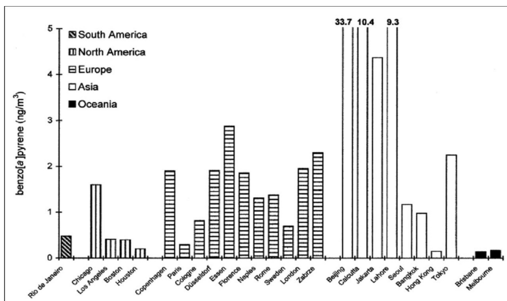
Figura 3. Níveis médios de benzo(a)pireno em ar ( \text{ng}\cdot\text{m}^{-3} ) para o Rio de Janeiro, cidades da América do Norte, Europa, Ásia e Oceania. (Fonte: Adaptado de Fernandes et al. 2002).
