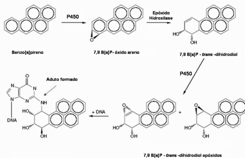
Figura 2. Esquema simplificado da ativação enzimática do benzo[a]pireno em diol epóxidos, na formação de adutos de DNA. Adaptado de Akcha et al. 2000.
