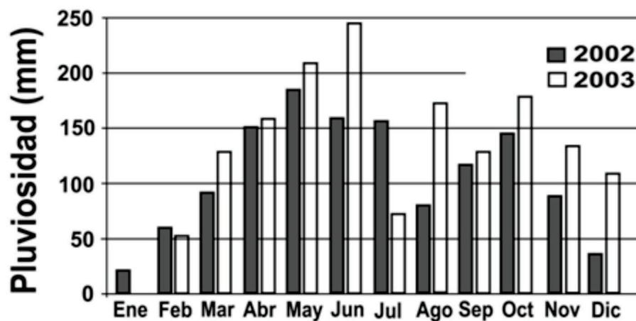
Figura 9. Variación de la pluviosidad durante los años 2002 y 2003 en el embalse Riogrande II. Figure 9. Variation of rainfall over the years 2002 and 2003 in the reservoir Riogrande II.
