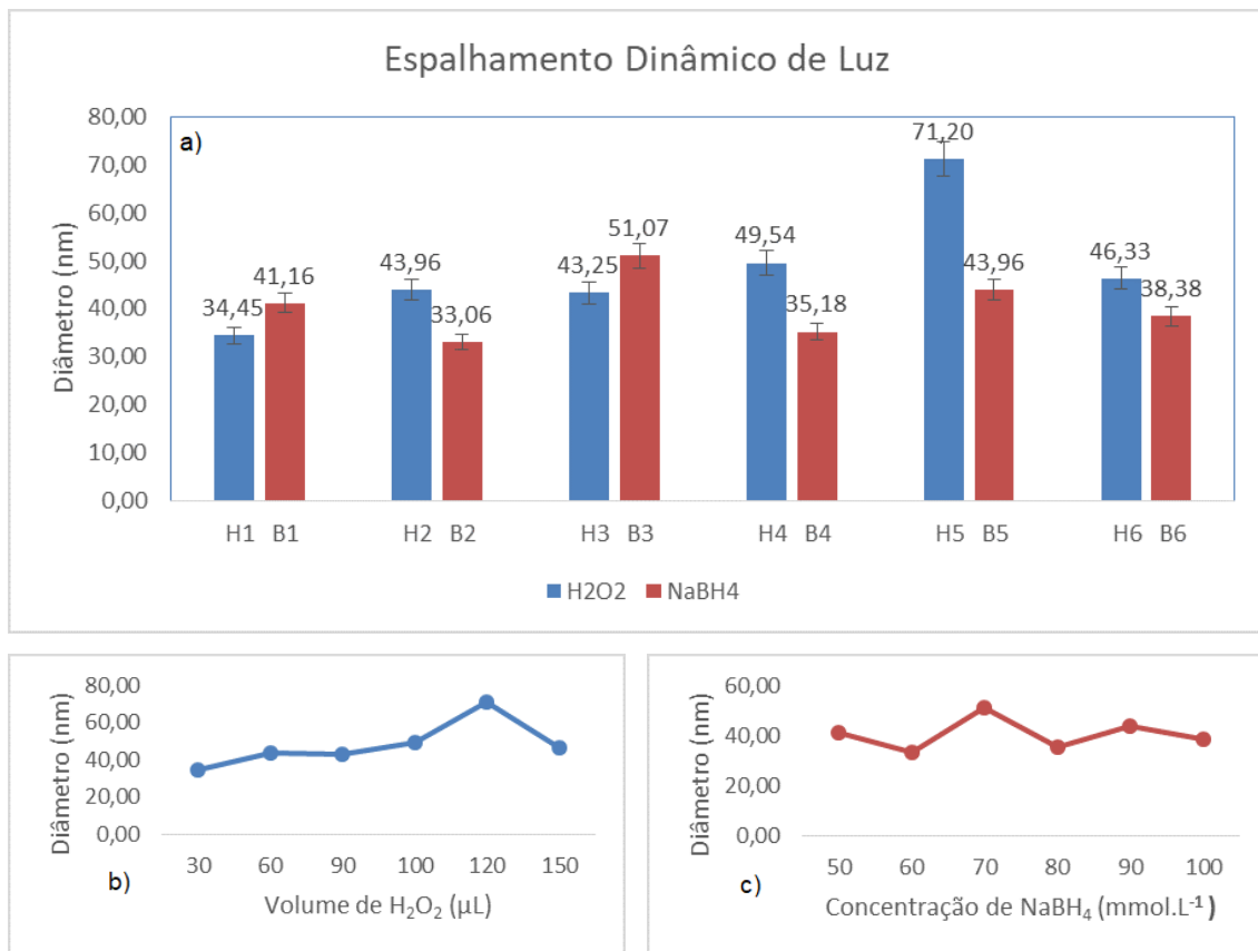
Figura 1: a) Comportamento do diâmetro hidrodinâmico das AgNPs em função da variação de NaBH 4 e H 2 O 2 . b) Linha de tendência do diâmetro hidrodinâmico em função do H 2 O 2 . c) Linha de tendência do diâmetro hidrodinâmico em função do NaBH 4 .
