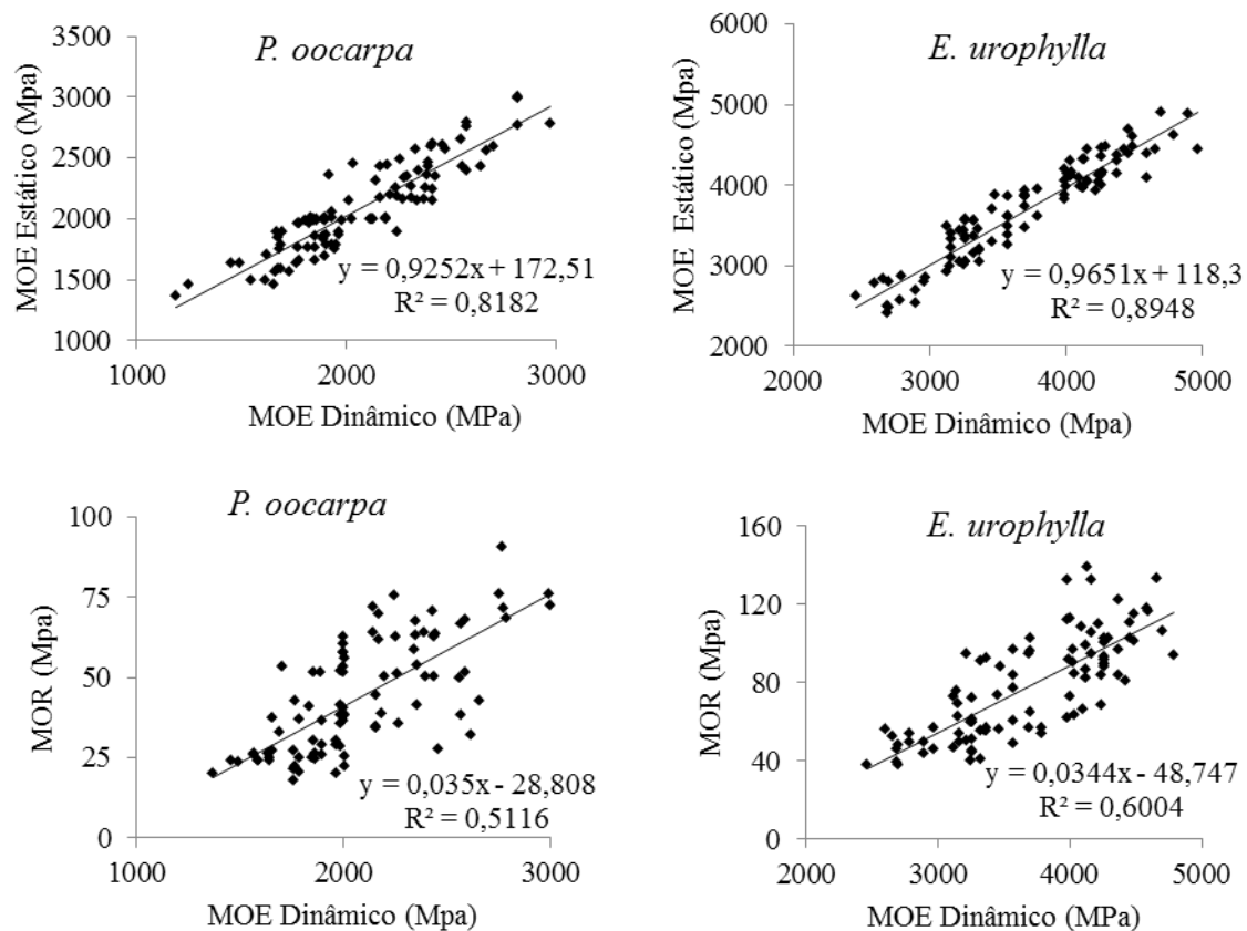
Figura 1: A correlação entre o módulo de elasticidade estático e módulo de ruptura com o módulo de elasticidade dinâmico medido pelo sistema BING na madeira termorretrificada de Eucalyptus urophylla e Pinus oocarpa .
