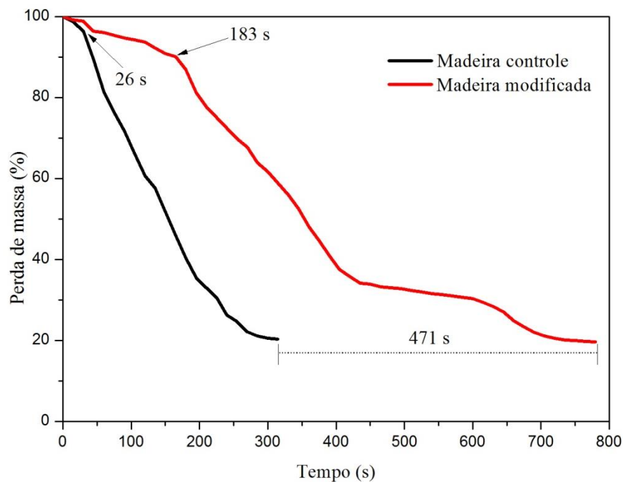
Figura 6: Comportamento das madeiras controle e modificada com TiO_2 por meio do método solvotermal assistido por micro-ondas no ensaio teste de retardamento de fogo
