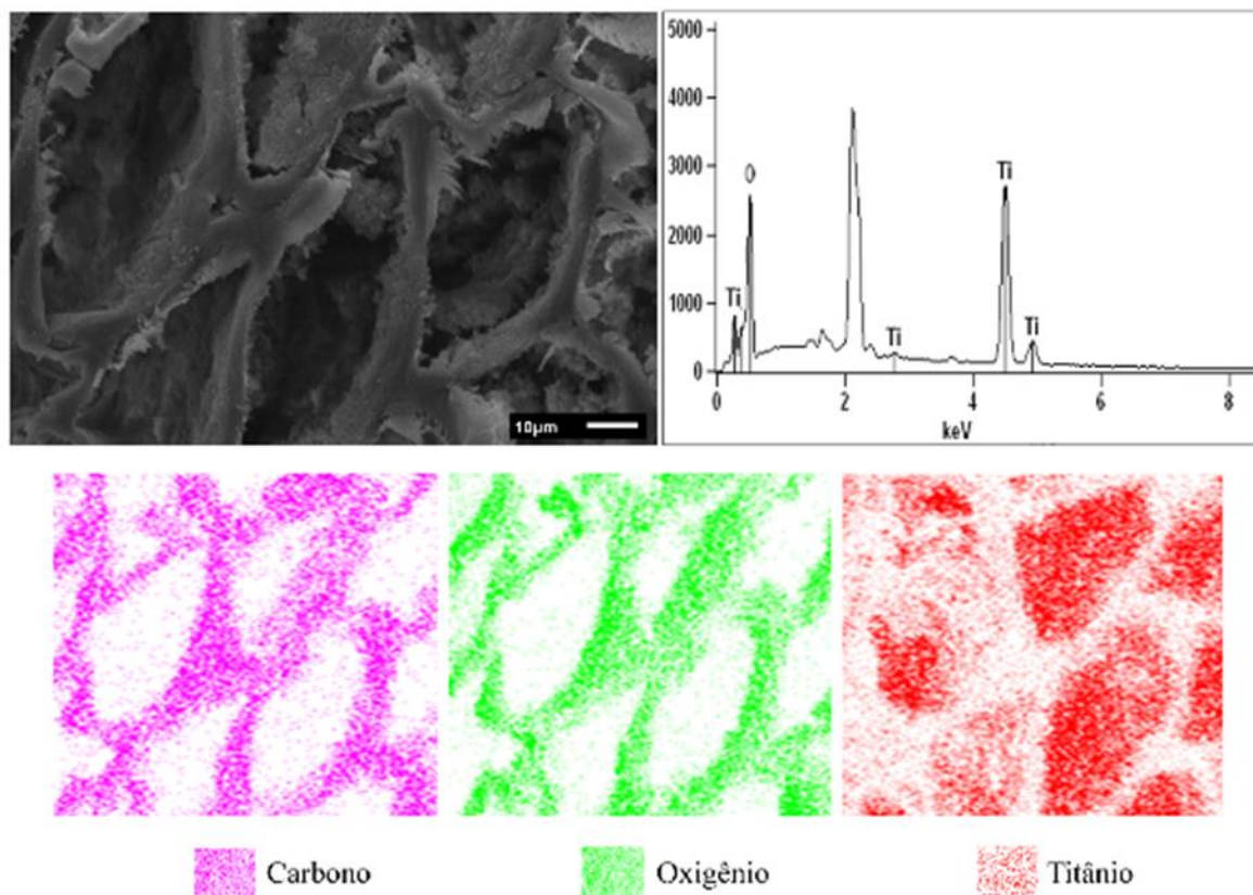
Figura 2: Espectro e mapeamento EDX na seção transversal da madeira modificada com TiO 2 por meio do método solvotermal assistido por micro-ondas.
