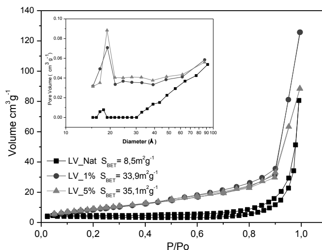
Figura 1: Isotermas de adsorção/dessorção de \text{N}_2 dos materiais usando o método BET a 77K.
