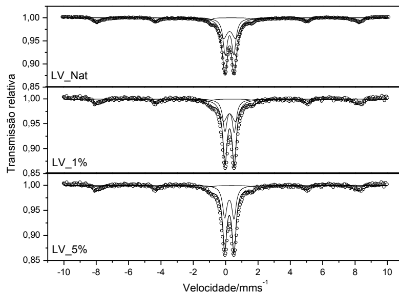
Figura 3: Espectros Mössbauer com fonte de ^{57}Co / Rh à temperatura ambiente, usando \alpha\text{-Fe} como referência.
