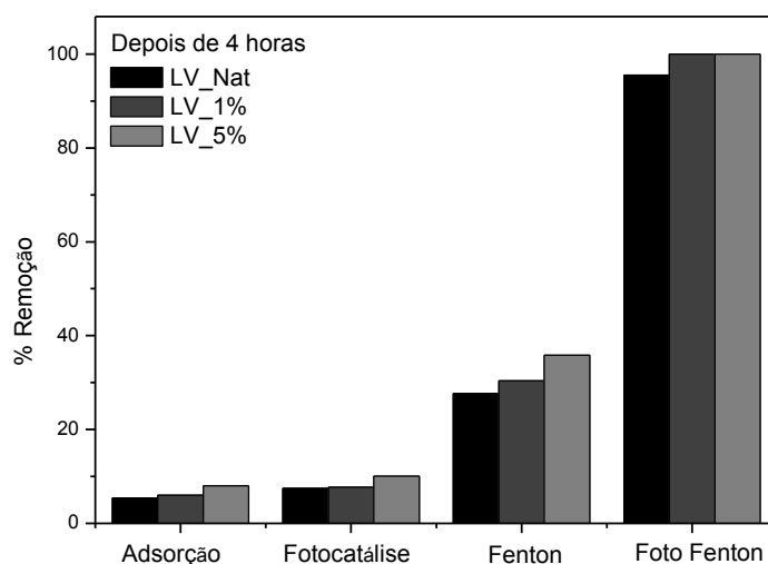
Figura 9: Comparação dos diferentes sistemas de remoção da molécula modelo de AM ( 10 \text{ mg L}^{-1} ).
