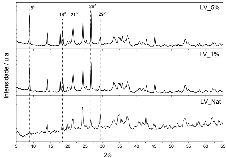
Figura 2: Difratoograma de raios X dos materiais usando radiação K\alpha Cu e varredura de 5 a 65° ( 2\theta ) a uma taxa de 1^\circ \text{min}^{-1}
