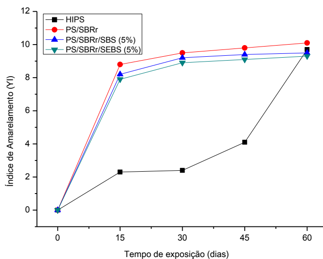
Figura 5: Evolução do índice de amarelamento (YI) do HIPS, da blenda PS/SBRr e das blendas compatibilizadas, submetidos ao envelhecimento termo-oxidativo.
