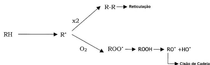
Figura 1: Reações básicas que levam às modificações da estrutura química de elastômeros [20].
