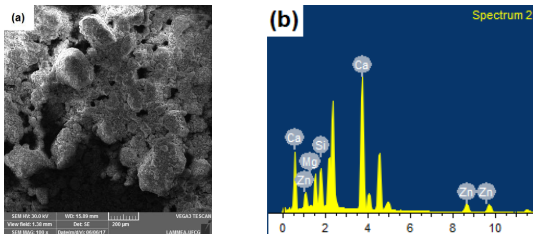
Figura 2. (a) Micrografia obtida por microscopia eletrônica de varredura (MEV) do pó calcinado da borracha reciclada; (b) Espectro de energia dispersiva (EDS) do pó sinterizado da borracha reciclada de SBRr.
