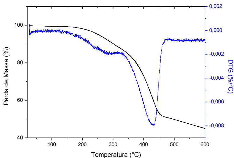
Figura 3: Curva TG/DTG do pó de borracha reciclada de SBRr, obtida sob atmosfera de N 2 , a 10°C/min e m = 5 mg.
