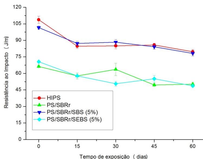
Figura 4: Resistência ao impacto do HIPS, da blenda PS/SBRr e das compatibilizadas submetidas ao envelhecimento termo-oxidativo.
