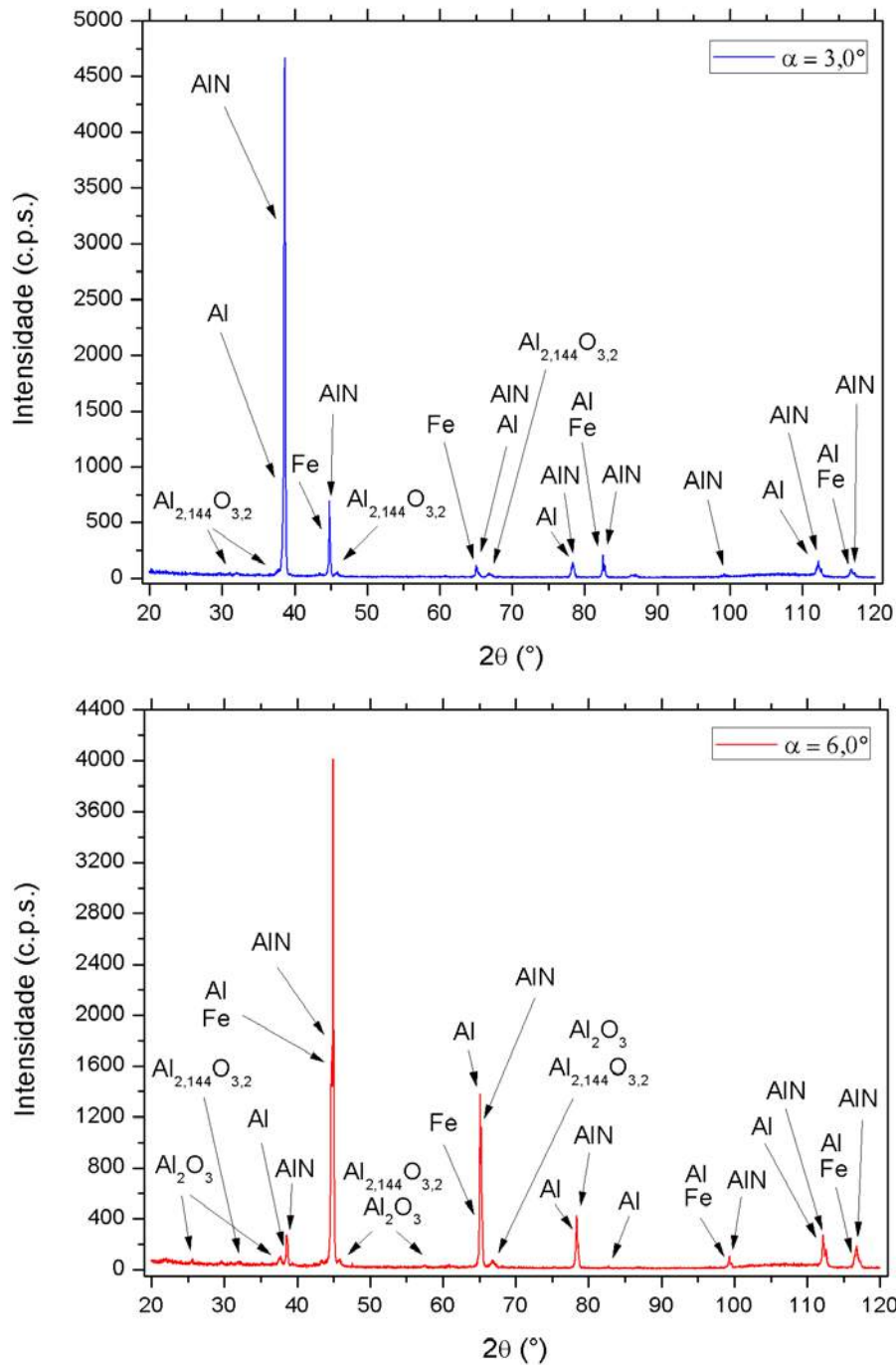
Figura 4: Difratogramas da amostra da liga Al-1,5%Fe tratada por RSL gerado por meio da técnica de DRXIR, a qual (a) com \alpha = 3^\circ e (b) \alpha = 6^\circ , ambas com radiação \text{Cu K}\alpha .
