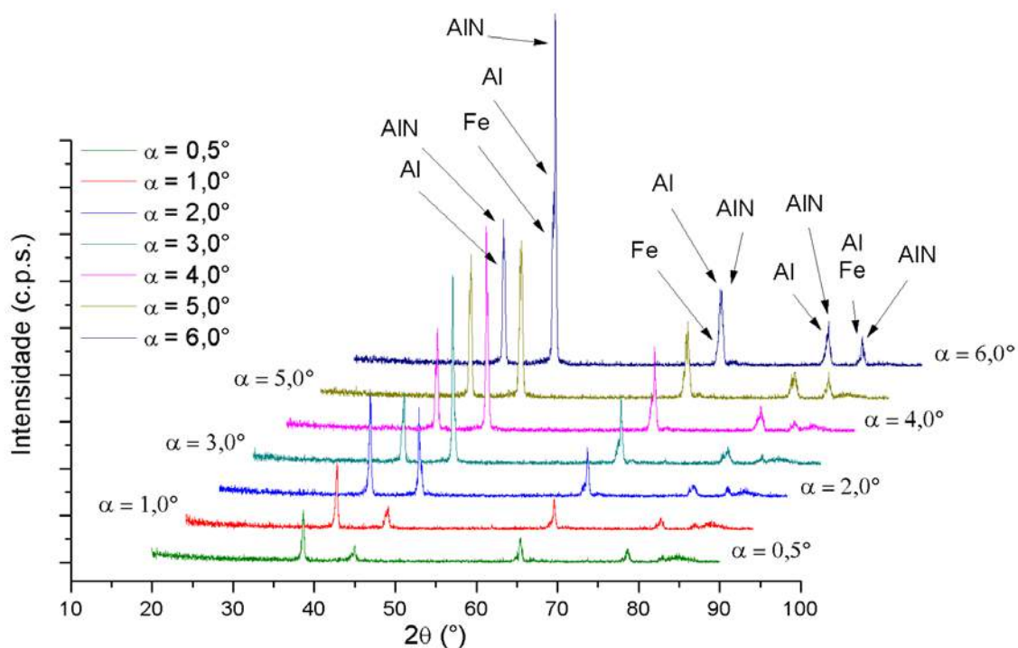
Figura 3: Difratogramas por meios da radiação \text{Cu K}\alpha aplicada na liga Al-1,5%Fe tratada por RSL. Com ângulo de incidência de \alpha=0,5^\circ , 1^\circ , 2^\circ , 3^\circ , 4^\circ , 5^\circ e 6^\circ .
