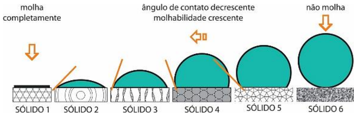
Figura 3: Esquema de diferentes ângulos de contato de uma gota d'água quando depositada sobre diferentes superfícies de sólidos. Fonte: DAPPER [14].)
