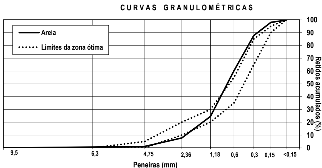
Figura 2: Curvas granulométricas da areia com limites da zona ótima padronizados [17].
