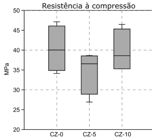
Figura 6: Gráficos de caixa para a compressão axial.
