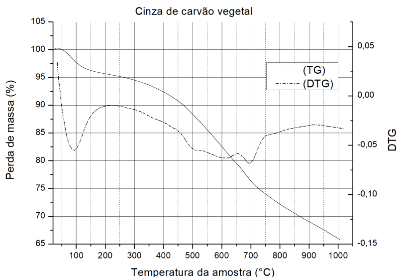
Figura 5: Curvas TG/DTG da CG.
