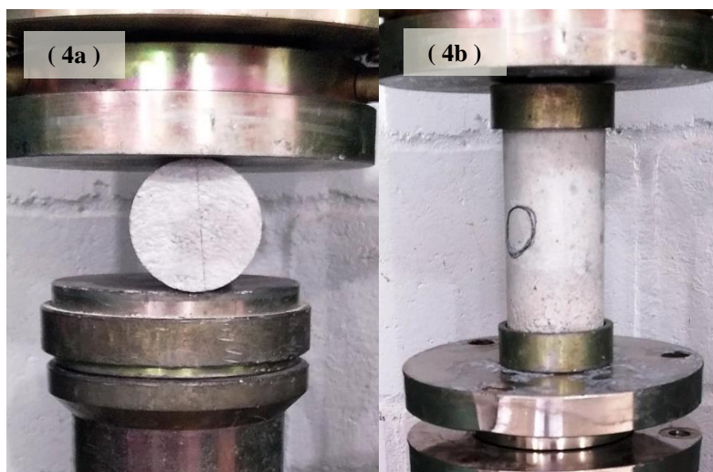
Figura 4: Preparação dos corpos de prova para compressão diametral (4a) e axial (4b).
