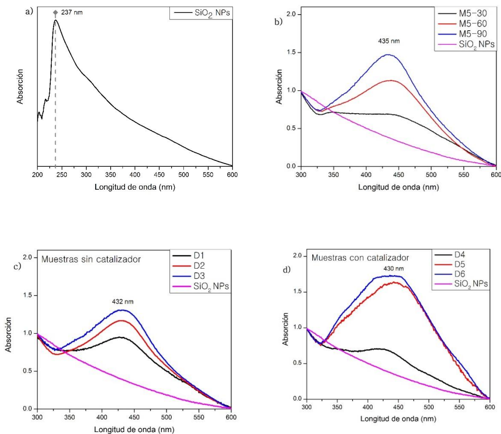
Figura 2. Espectros de absorción óptica de NPs SiO 2 antes (a) y después ser decoradas con NPs Ag mediante fotodeposición (b) y agitación (c y d).
