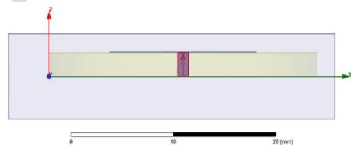
Figura 9: Porta de excitação da antena patch ( Lumped Port ).
