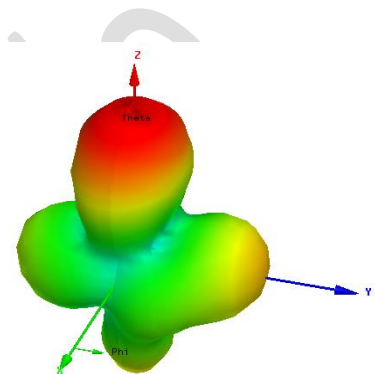
Figura 13: Diretividade da antena patch .
