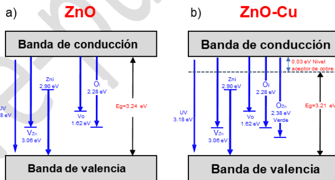
Figura 6: Diagrama de la estructura de bandas de películas delgadas de ZnO y ZnO-Cu.
