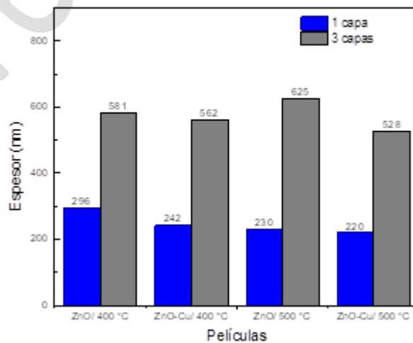
Figura 10: Espesor de películas de ZnO y ZnO-Cu tratadas térmicamente a 400 y 500°C
