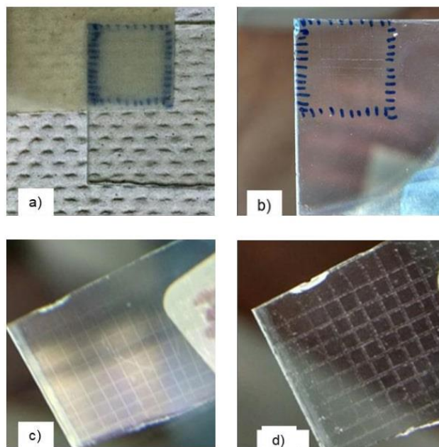
Figura 11: a) Película de ZnO con cinta adherida, b) película de ZnO después de la prueba de la adherencia, c) película de ZnO-Cu con la retícula marcada antes de colocar la cinta, d) película de ZnO-Cu después de la prueba de adherencia
