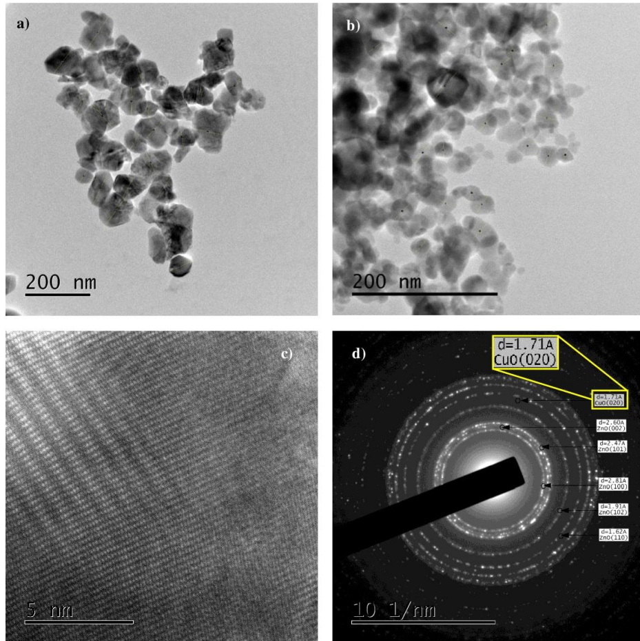
Figura 7: Imágenes TEM de (a) nanopartículas de ZnO (b) y ZnO-Cu obtenidas a 400 °C, (c) arreglo atómico de ZnO y (d) SAED de película delgada de ZnO-Cu en donde se observa la difracción de CuO.
