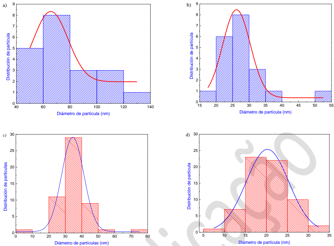
Figura 9: Histograma de nanopartículas de ZnO (a y c) y ZnO dopado con Cobre (b y d) a 400 y 500 °C.
