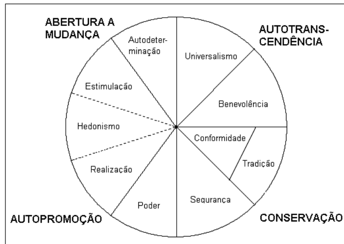
Figura 2: Estrutura teórica da relação entre valores. Fonte: Inventário de Valores de Schwartz (SVS) - 1992
