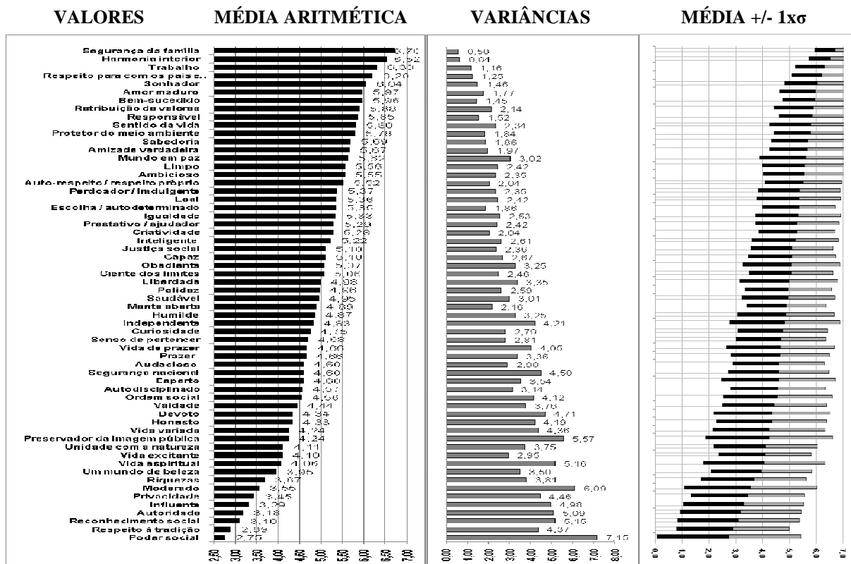
Gráfico 2: Hierarquia dos Valores da empresa conforme Schwartz (1992) e correlação com \sigma^2 e com \pm 1\sigma .
